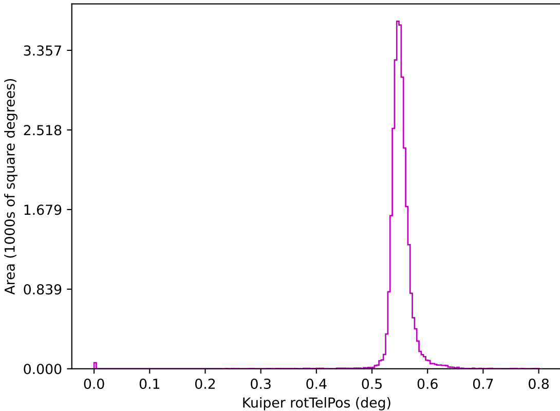
too_10_4v3.4_10yrs z: Kuiper rotTelPos
