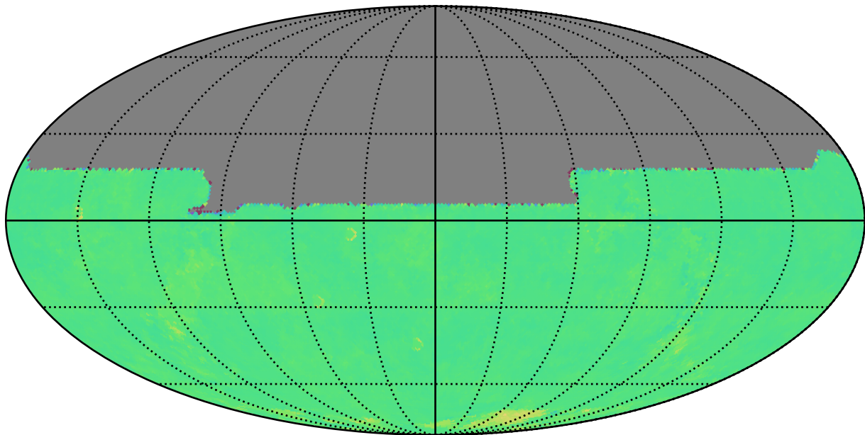
too_10_4v3.4_10yrs y: Kuiper rotTelPos
