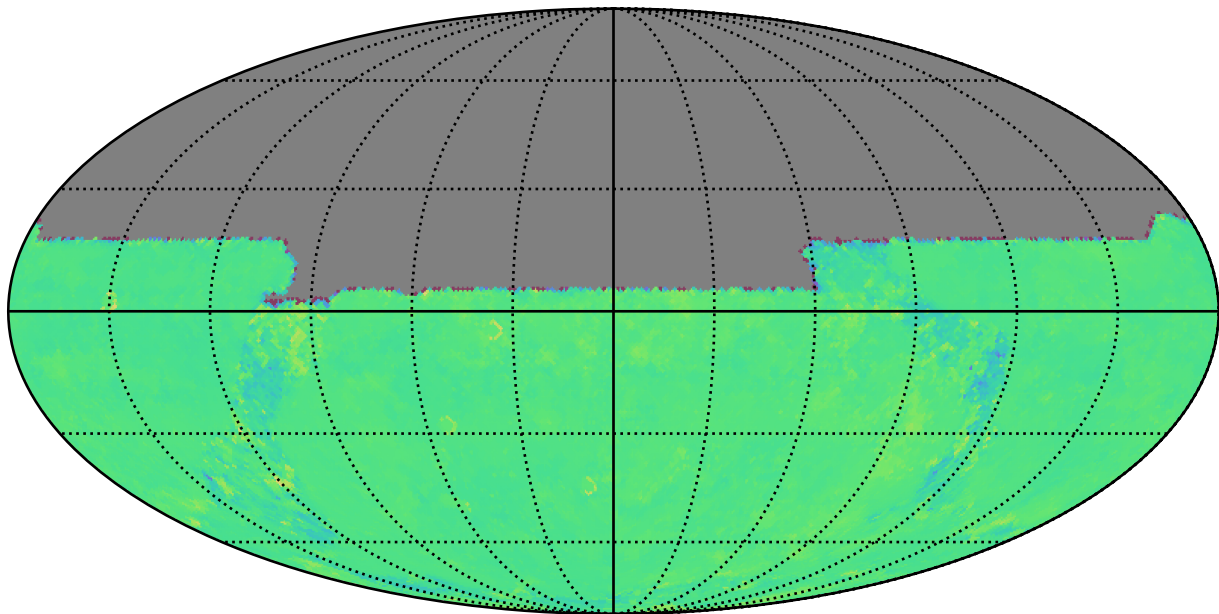
too_10_4v3.4_10yrs u: Kuiper rotTelPos
