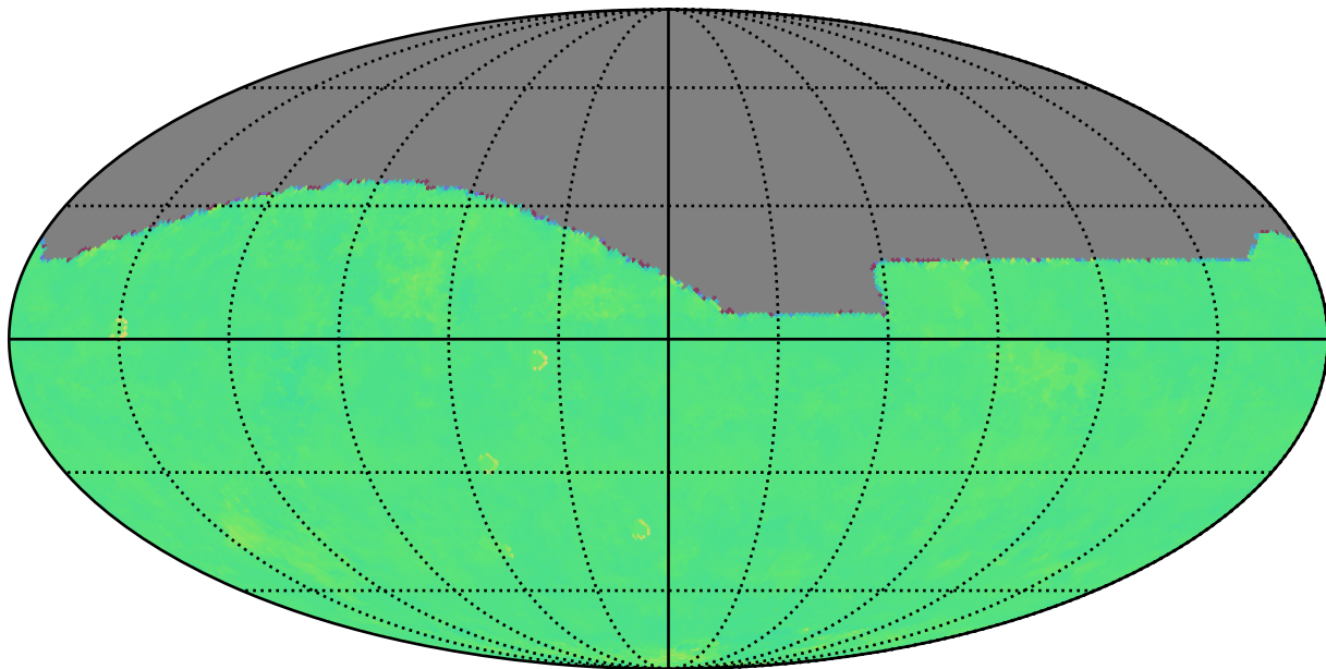
too_10_4v3.4_10yrs i: Kuiper rotTelPos
