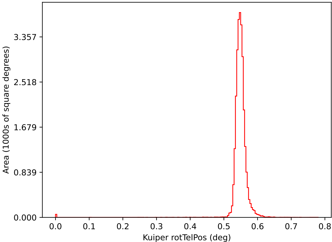
too_10_4v3.4_10yrs i: Kuiper rotTelPos
