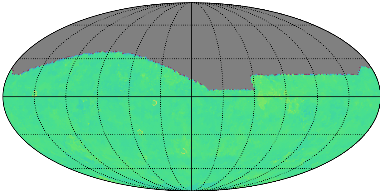
too_10_4v3.4_10yrs g: Kuiper rotTelPos
