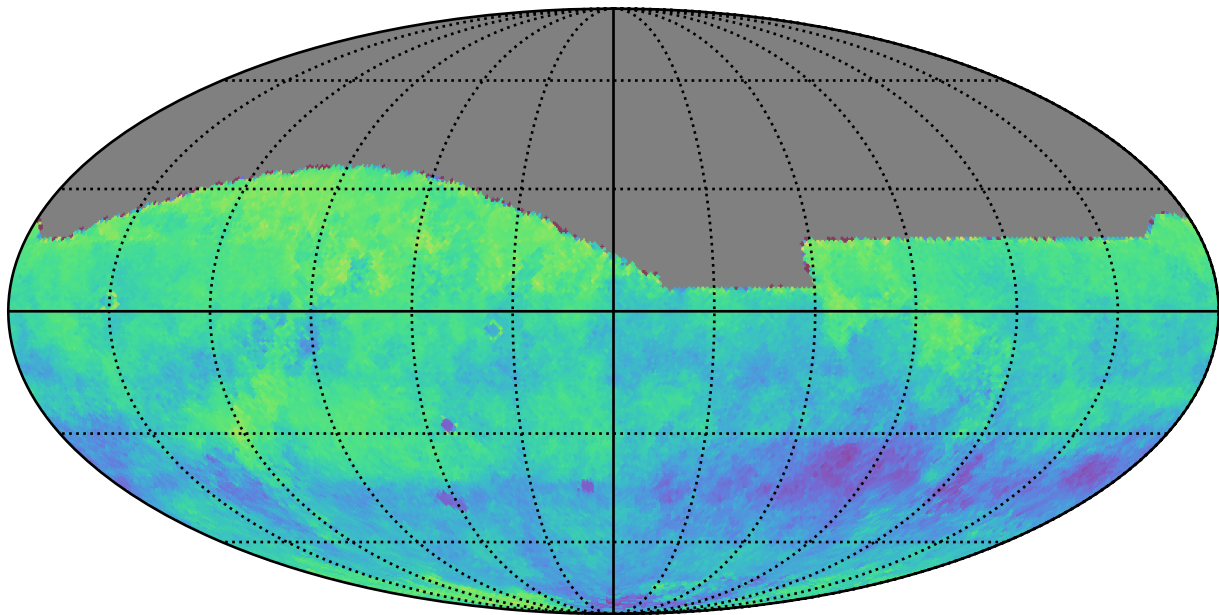
too_10_4v3.4_10yrs z: Kuiper rotSkyPos
