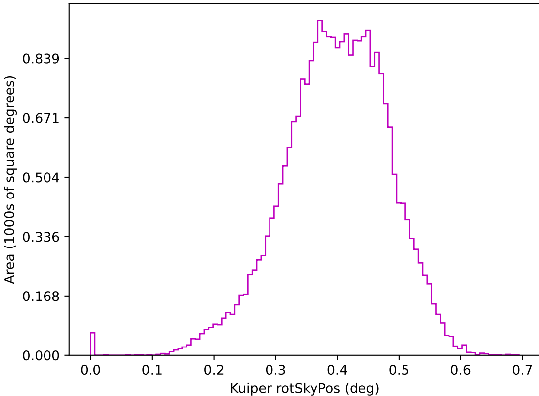
too_10_4v3.4_10yrs z: Kuiper rotSkyPos
