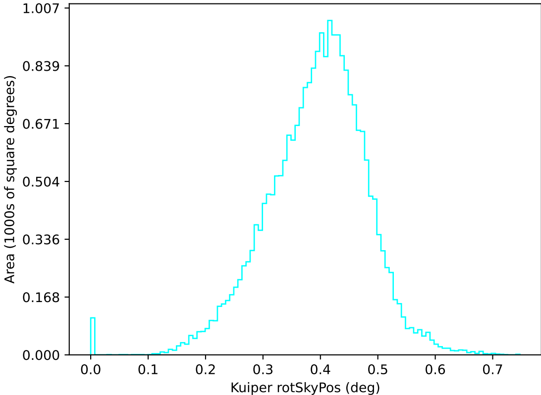
too_10_4v3.4_10yrs u: Kuiper rotSkyPos
