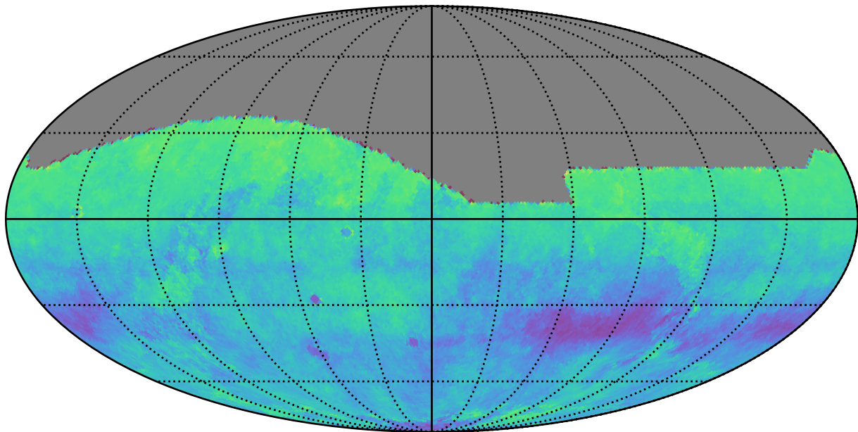
too_10_4v3.4_10yrs r: Kuiper rotSkyPos
