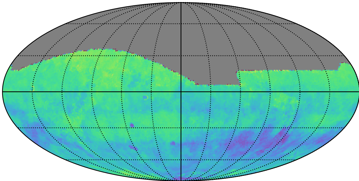
too_10_4v3.4_10yrs i: Kuiper rotSkyPos
