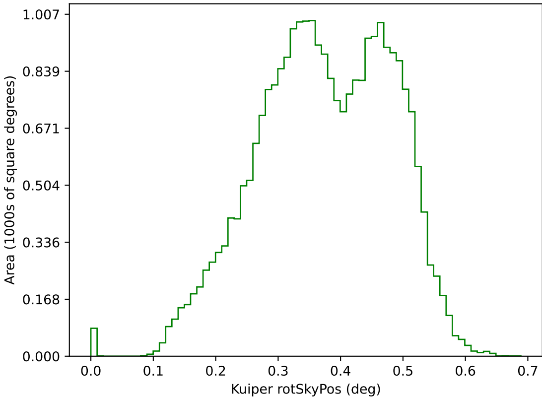
too_10_4v3.4_10yrs g: Kuiper rotSkyPos
