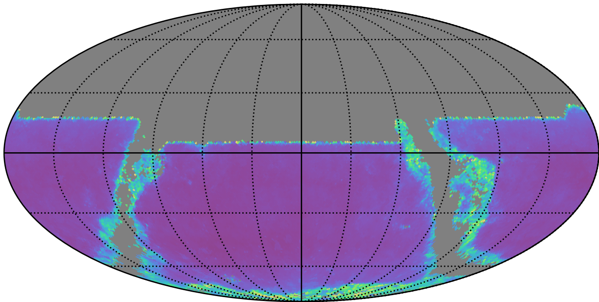
too_10_4v3.4_10yrs y band: AGN SF_uncert
