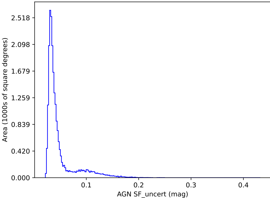
too_10_4v3.4_10yrs y band: AGN SF_uncert
