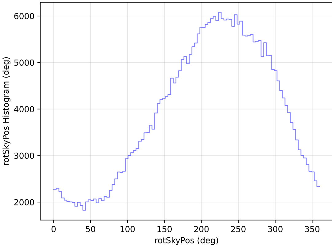
too_10_4v3.4_10yrs WFD y band: rotSkyPos Histogram
