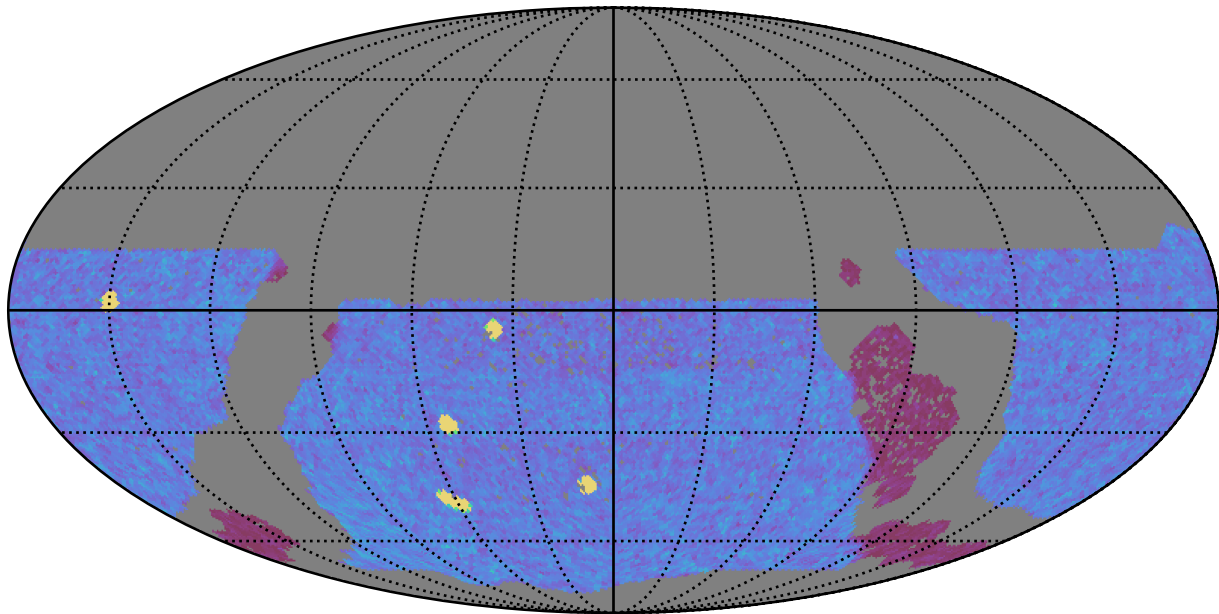
too_10_4v3.4_10yrs WFD y band: NVisits
