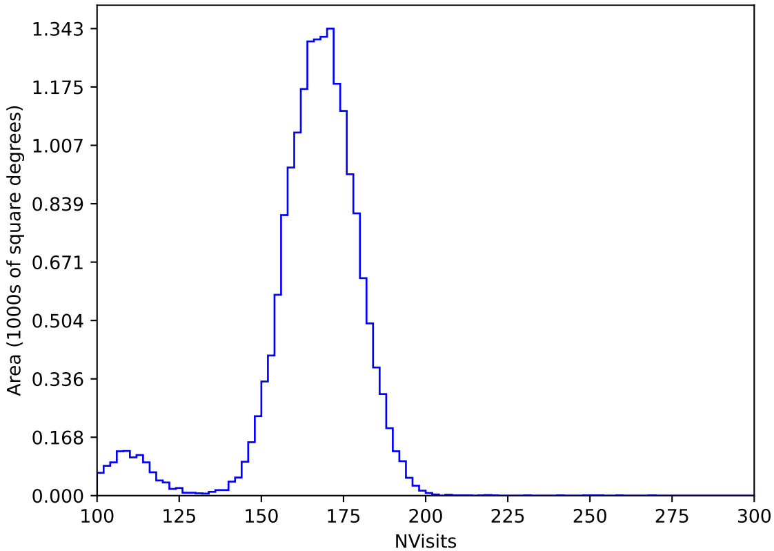
too_10_4v3.4_10yrs WFD y band: NVisits
