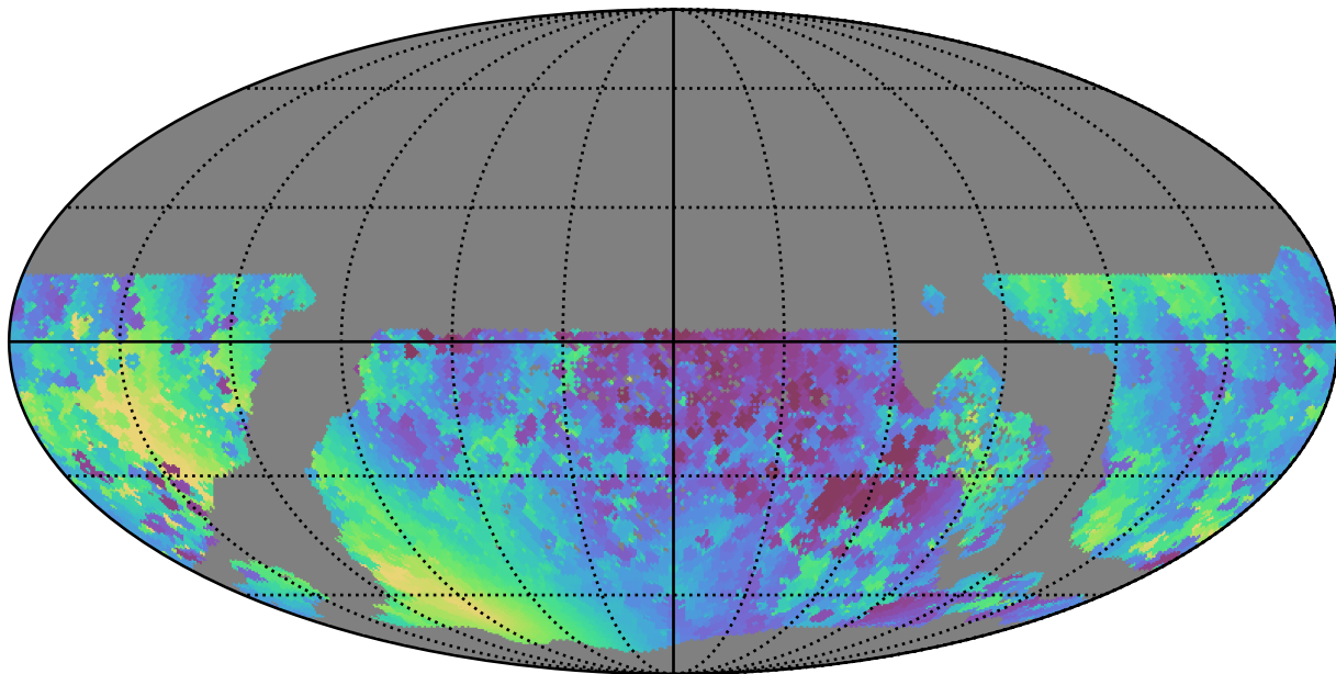
too_10_4v3.4_10yrs WFD y band: Min solarElong
