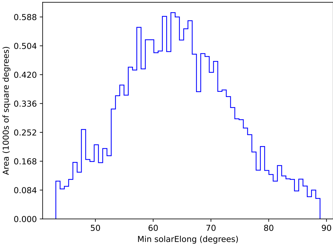
too_10_4v3.4_10yrs WFD y band: Min solarElong
