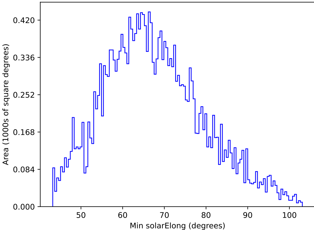
too_10_4v3.4_10yrs All sky y band: Min solarElong
