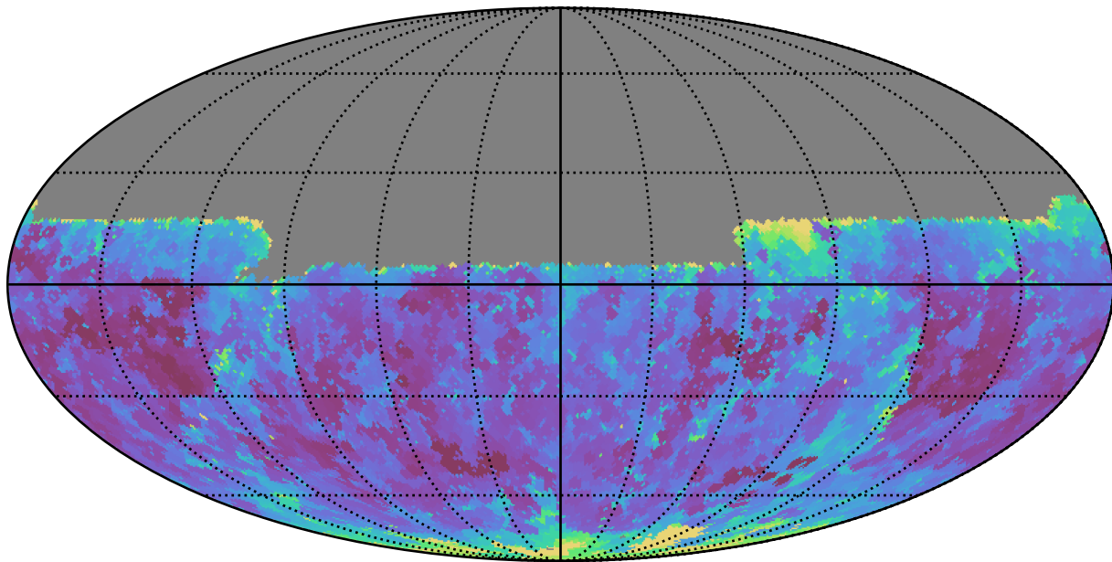
too_10_4v3.4_10yrs Yr 1 y band: Min seeingGeom
