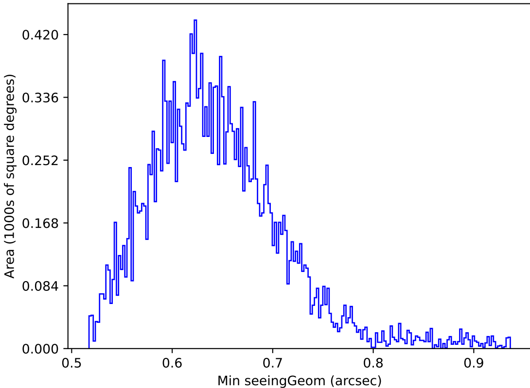
too_10_4v3.4_10yrs Yr 1 y band: Min seeingGeom
