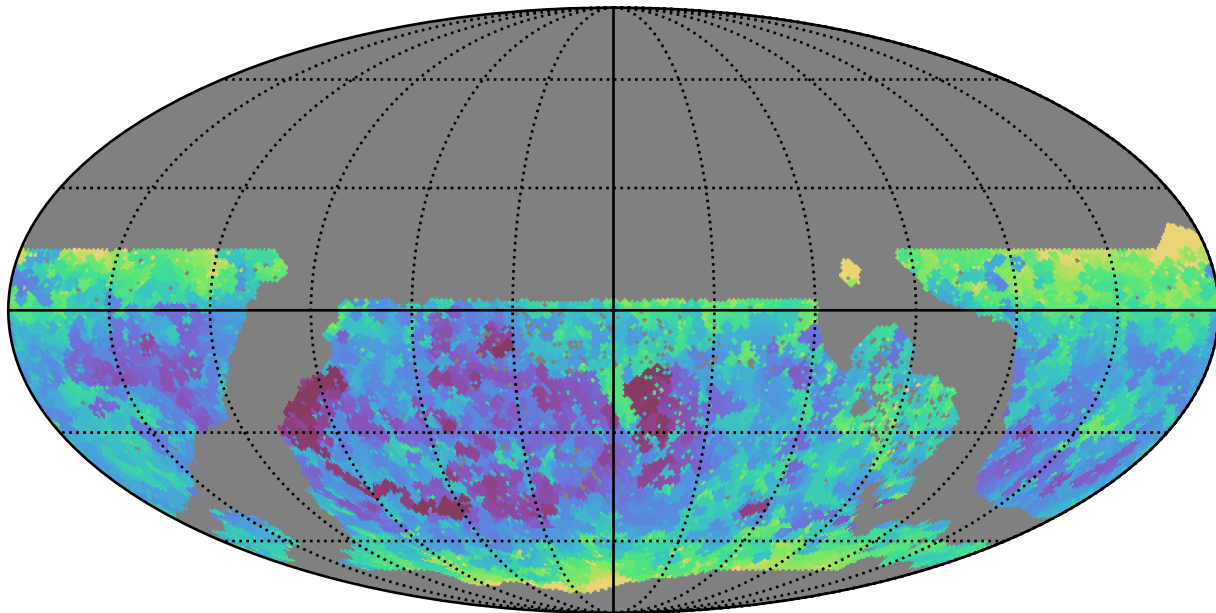
too_10_4v3.4_10yrs WFD y band: Min seeingEff
