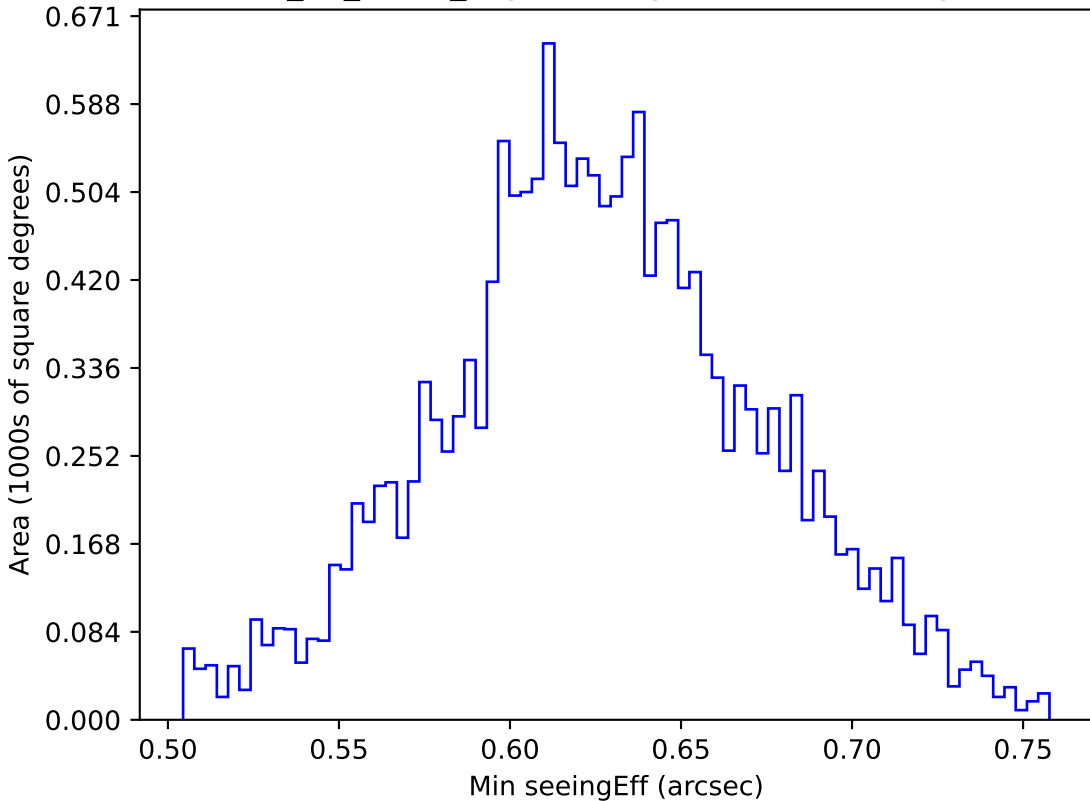
too_10_4v3.4_10yrs WFD y band: Min seeingEff
