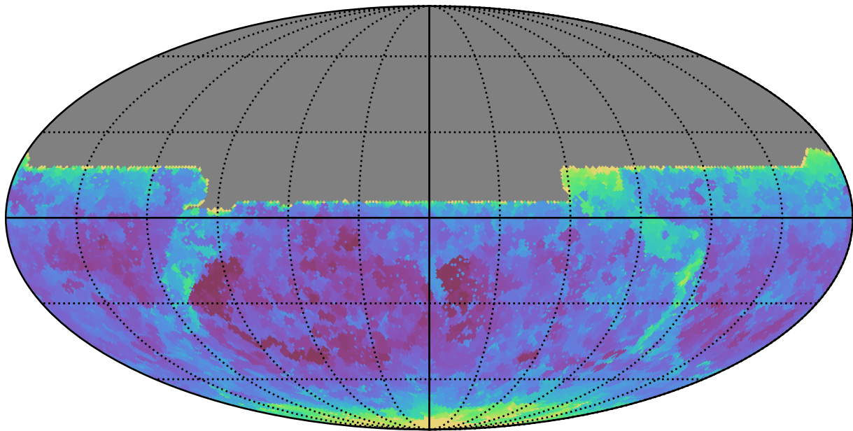
too_10_4v3.4_10yrs All sky y band: Min seeingEff
