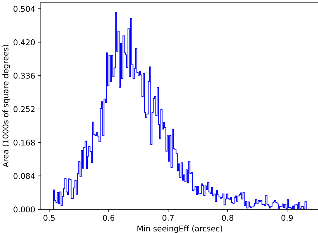
too_10_4v3.4_10yrs All sky y band: Min seeingEff
