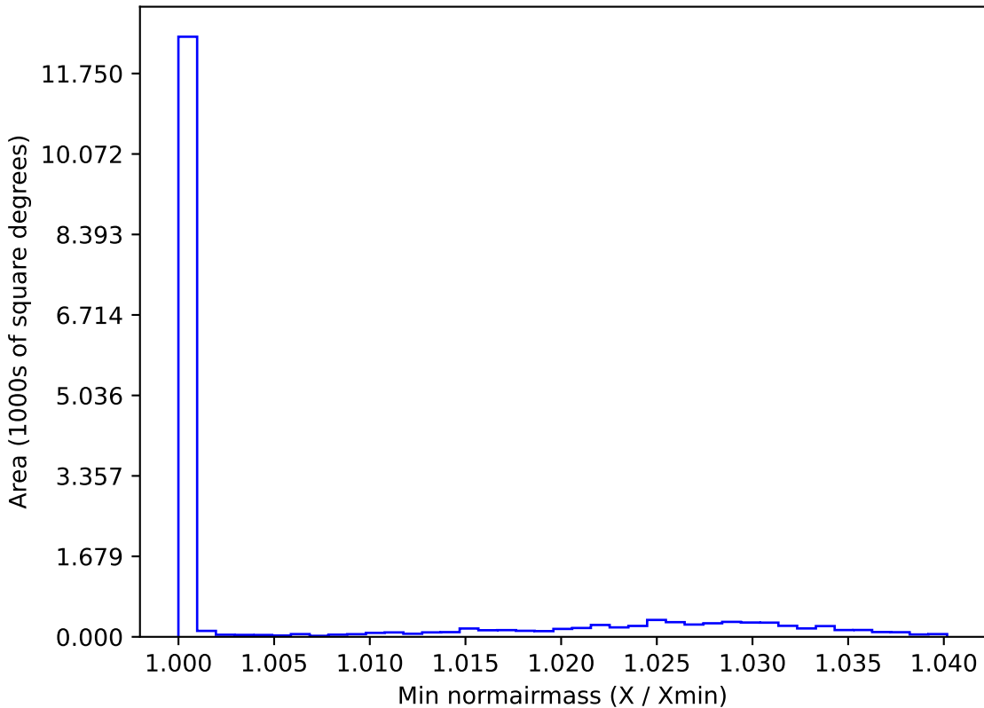
too_10_4v3.4_10yrs WFD y band: Min normairmass
