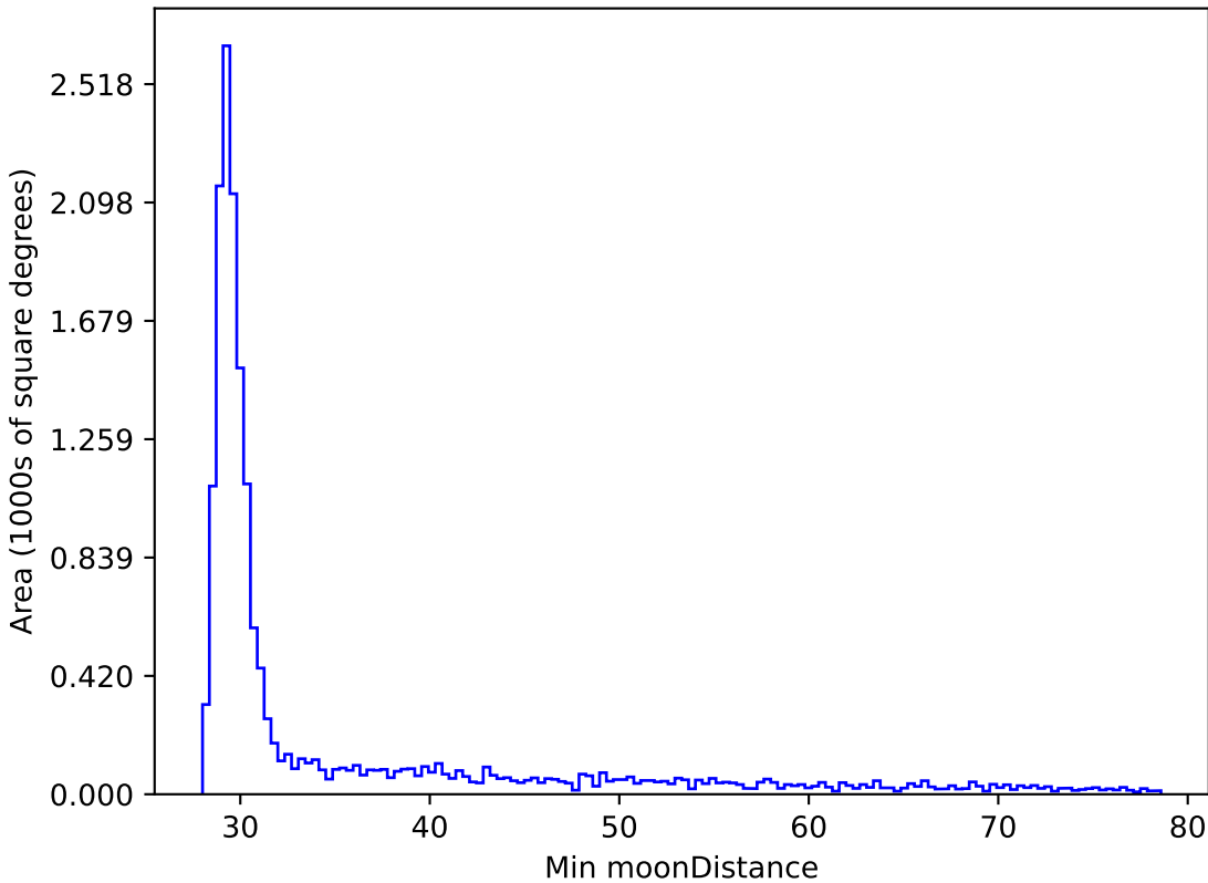
too_10_4v3.4_10yrs WFD y band: Min moonDistance
