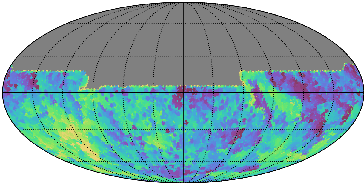
too_10_4v3.4_10yrs All sky y band: Min fiveSigmaDepth
