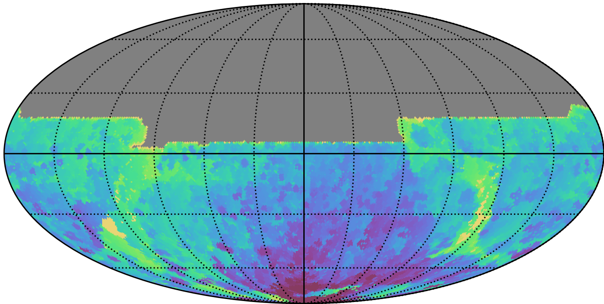
too_10_4v3.4_10yrs All sky y band: Min HA
