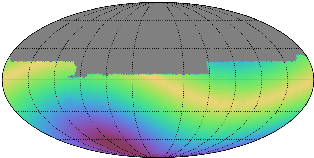
too_10_4v3.4_10yrs All sky y band: Max solarElong
