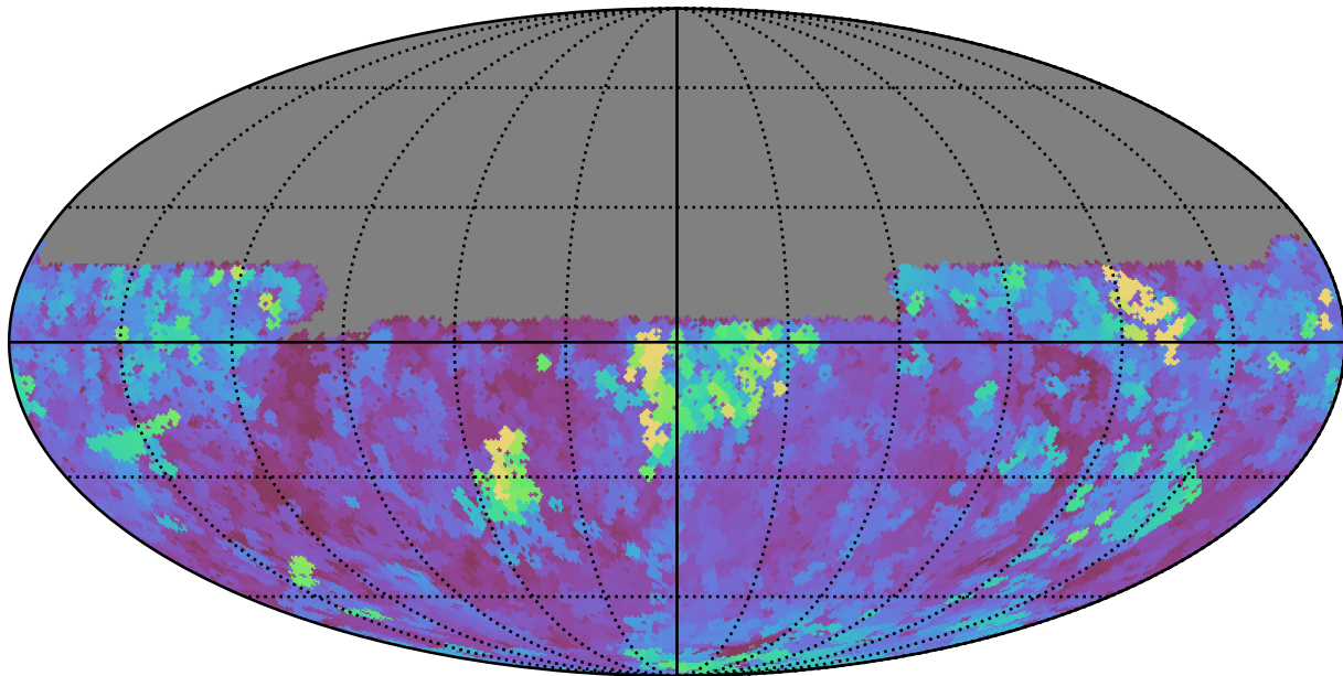
too_10_4v3.4_10yrs Yr 1 y band: Max seeingGeom
