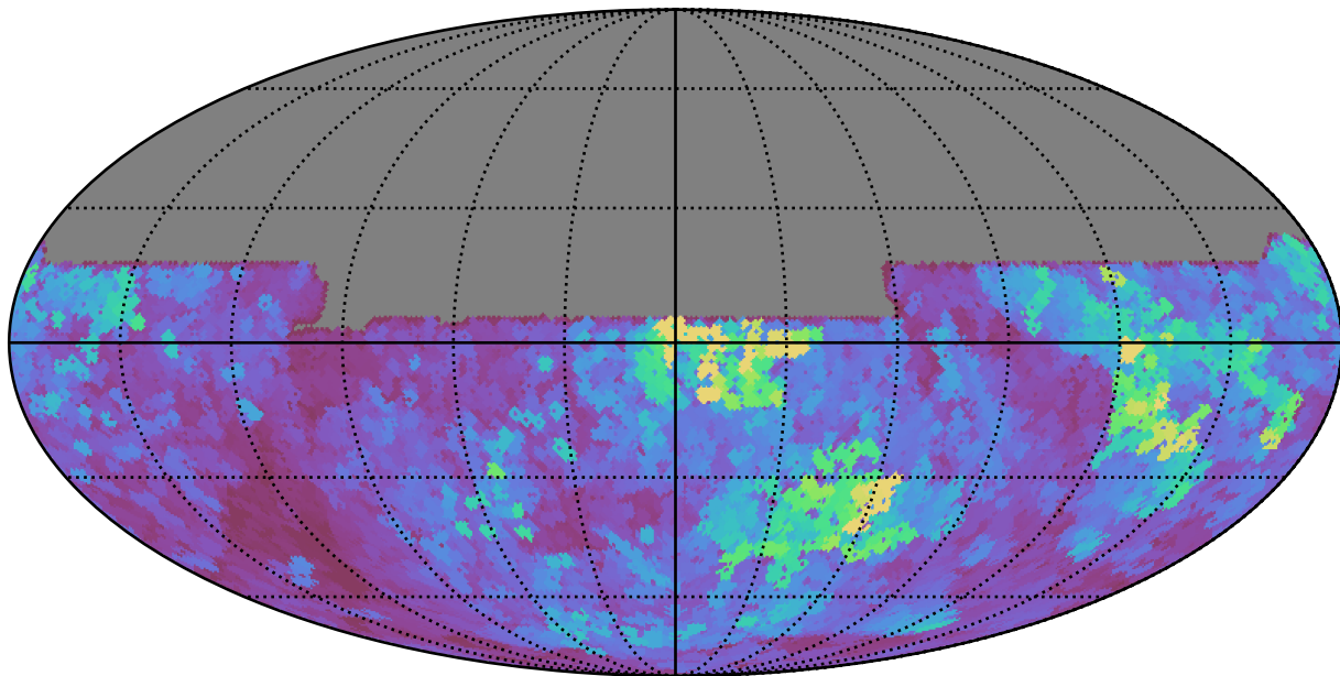
too_10_4v3.4_10yrs All sky y band: Max seeingEff
