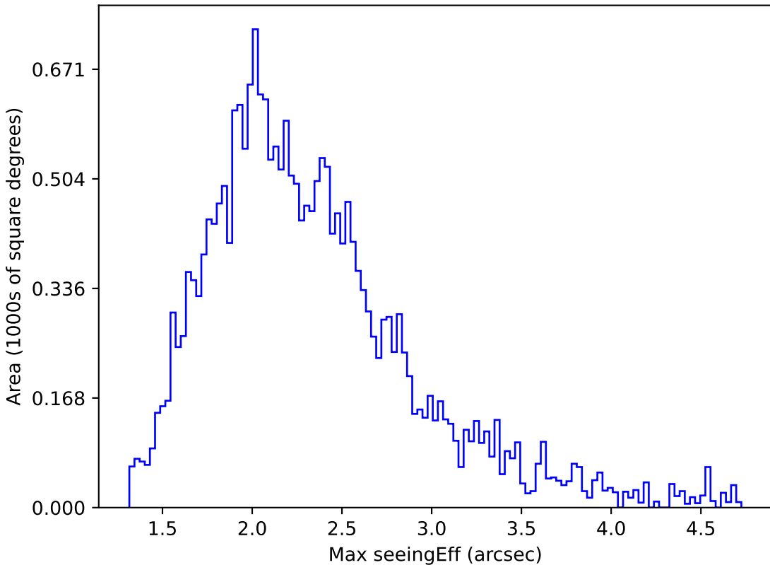
too_10_4v3.4_10yrs All sky y band: Max seeingEff
