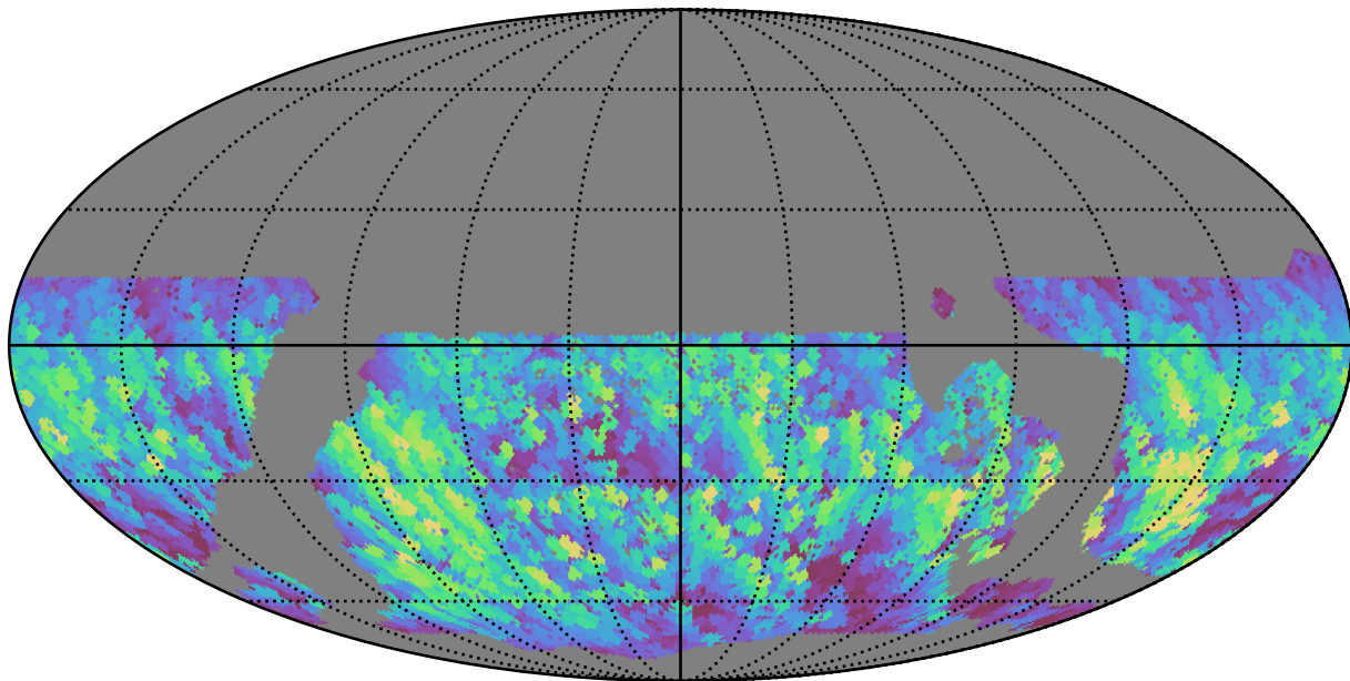
too_10_4v3.4_10yrs WFD y band: Max normairmass
