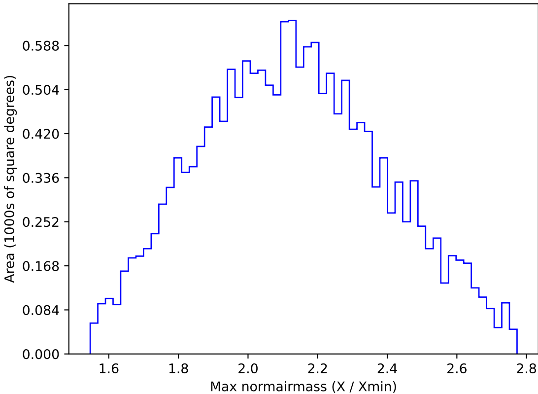
too_10_4v3.4_10yrs WFD y band: Max normairmass
