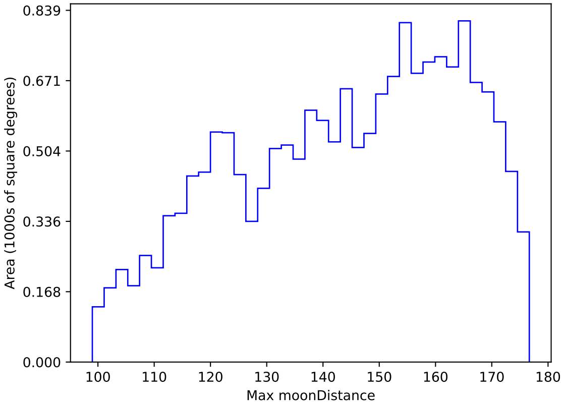
too_10_4v3.4_10yrs WFD y band: Max moonDistance
