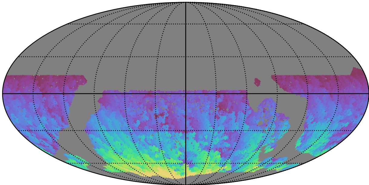
too_10_4v3.4_10yrs WFD y band: Max HA
