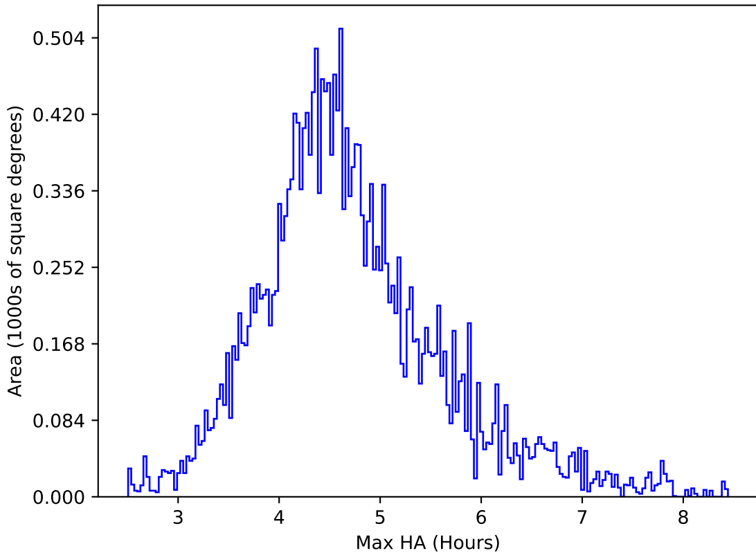
too_10_4v3.4_10yrs All sky y band: Max HA
