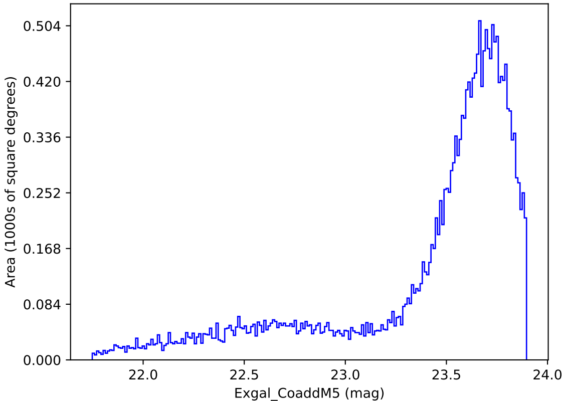
too_10_4v3.4_10yrs Yr 1 y band: Exgal_CoaddM5
