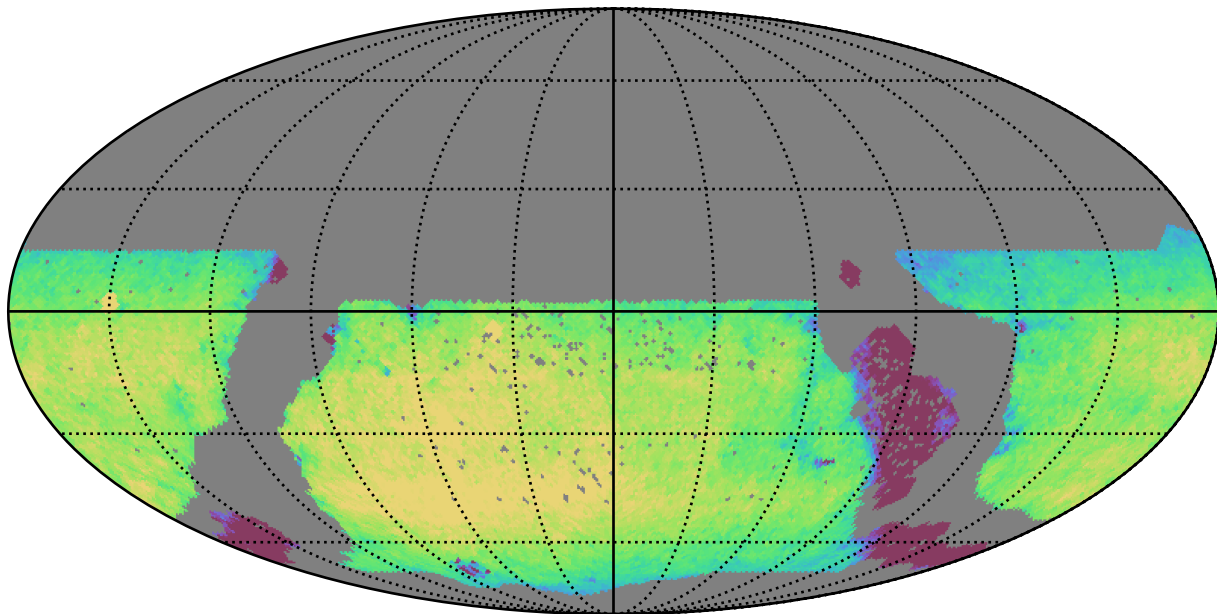
too_10_4v3.4_10yrs WFD y band: Exgal_CoaddM5
