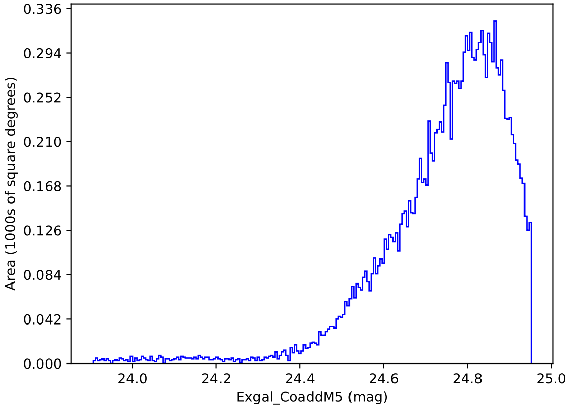
too_10_4v3.4_10yrs WFD y band: Exgal_CoaddM5
