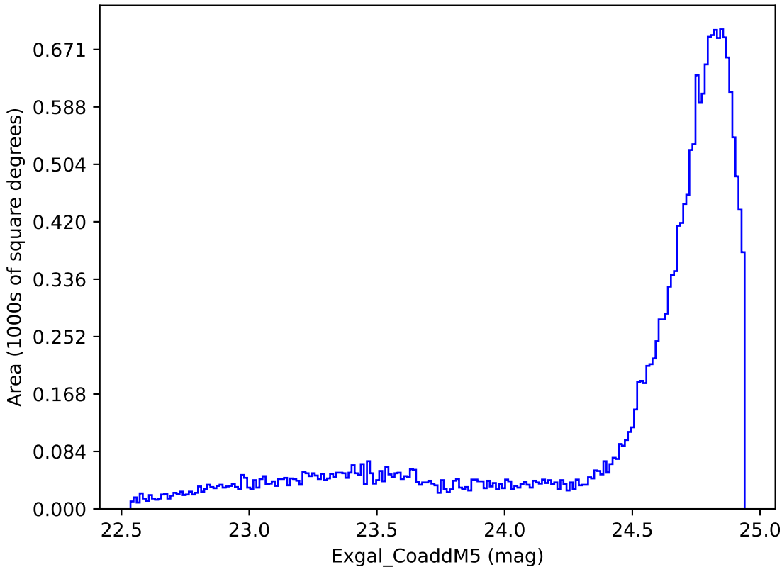
too_10_4v3.4_10yrs All sky y band: Exgal_CoaddM5
