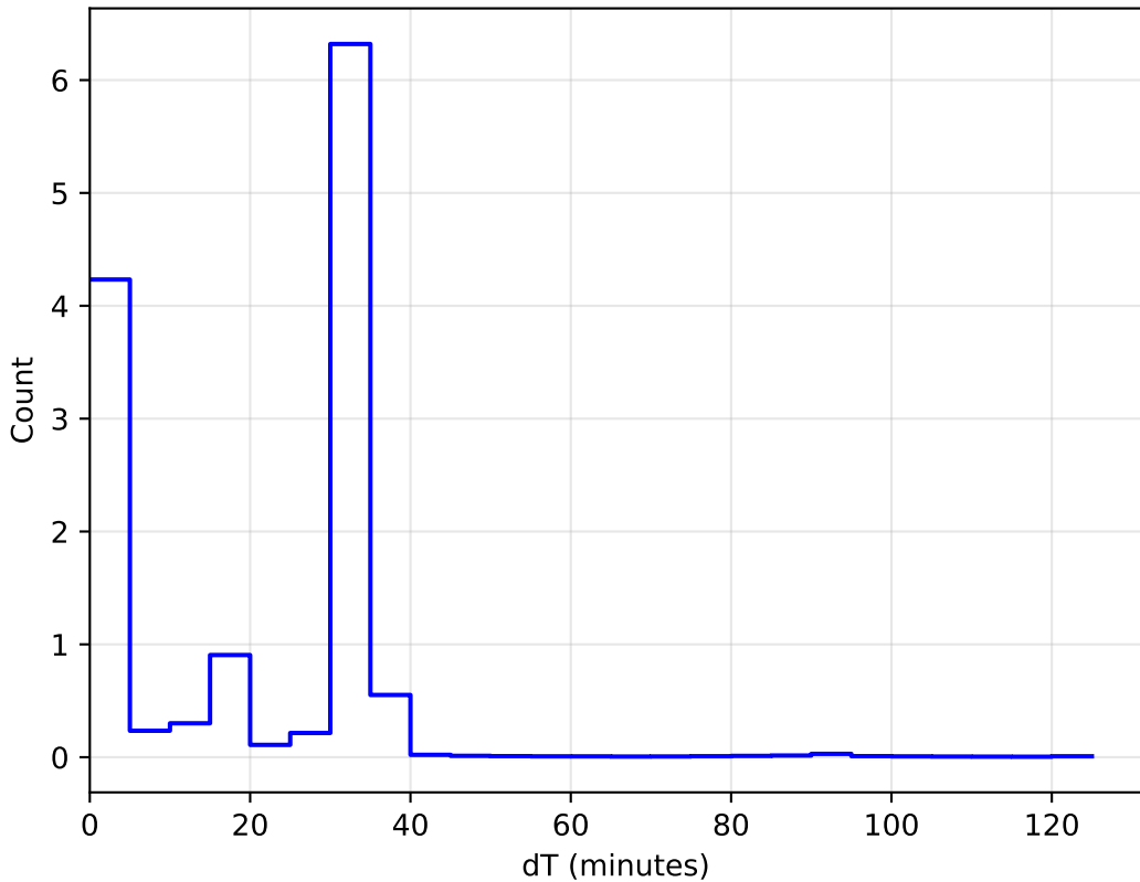
1e6 too_10_4v3.4_10yrs All sky: DeltaT Histogram
