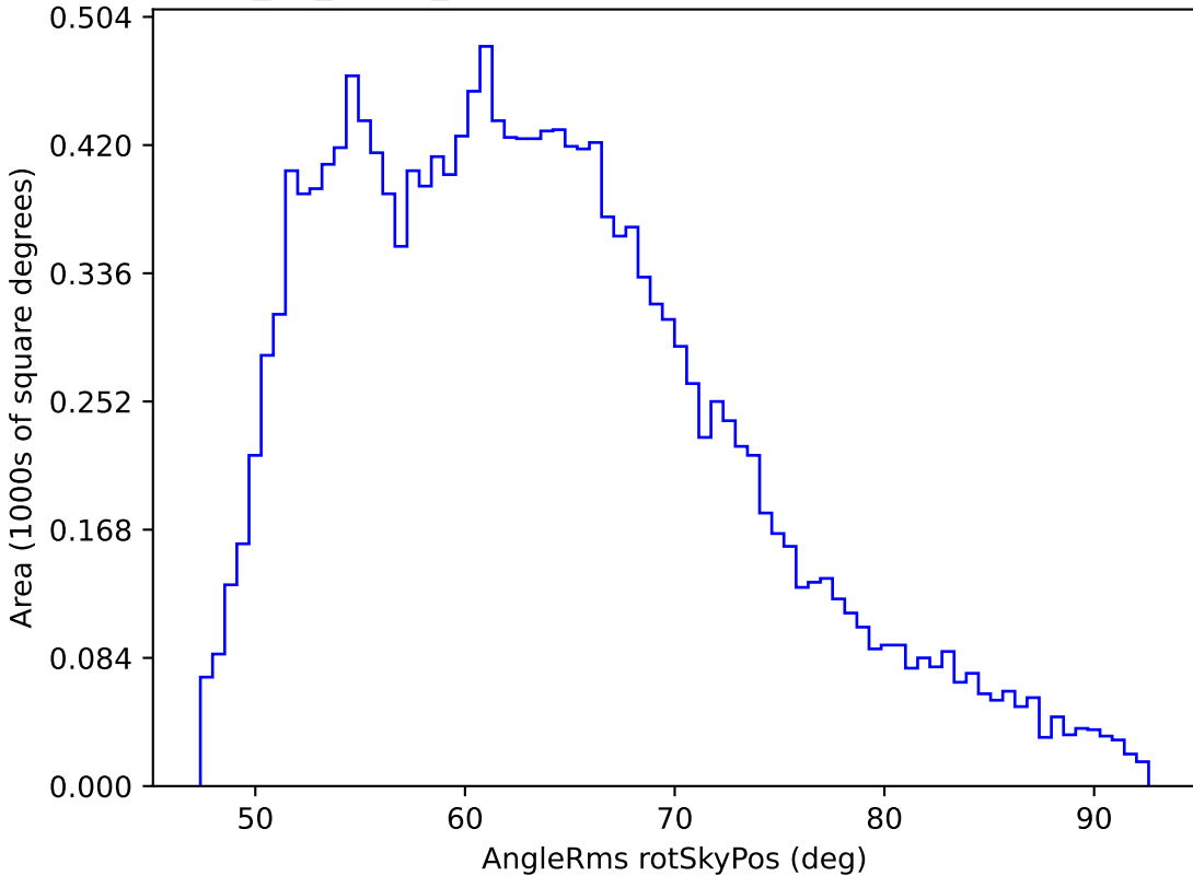
too_10_4v3.4_10yrs WFD y band: AngleRms rotSkyPos
