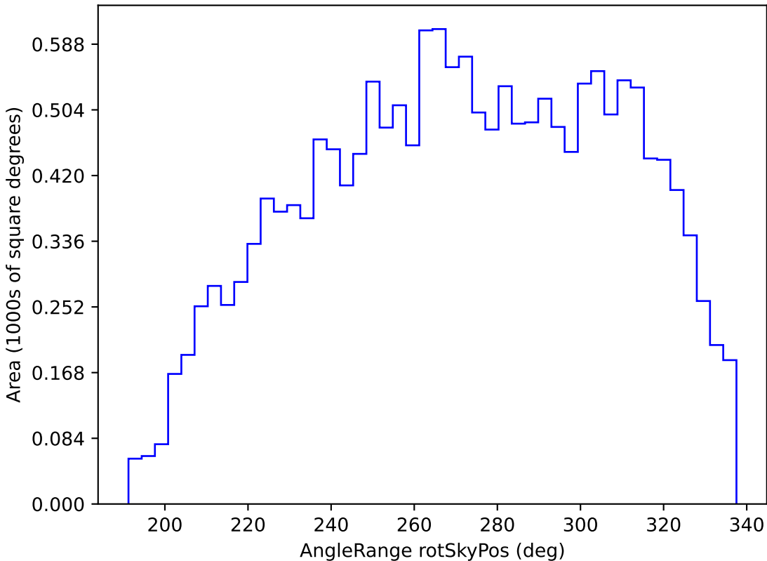
too_10_4v3.4_10yrs WFD y band: AngleRange rotSkyPos
