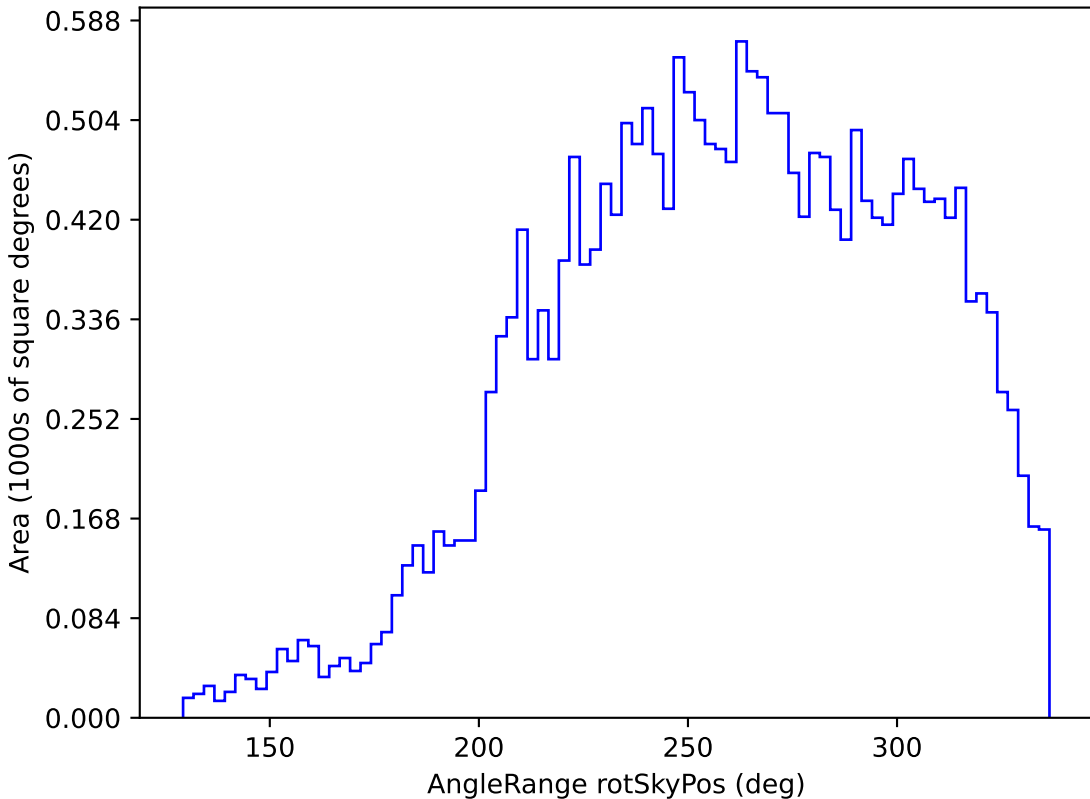
too_10_4v3.4_10yrs All sky y band: AngleRange rotSkyPos
