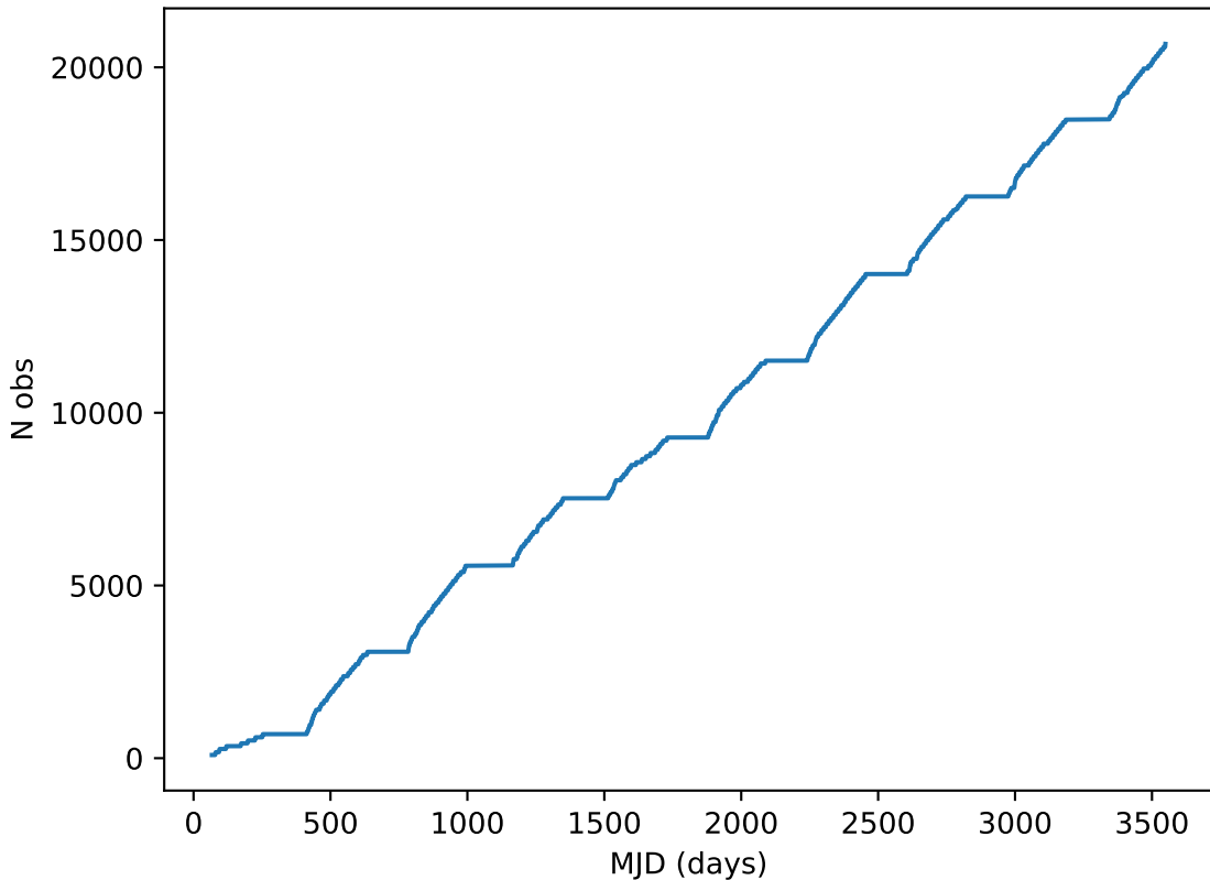
too_10_4v3.4_10yrs note like DD:ELAISS1%: Cumulative
