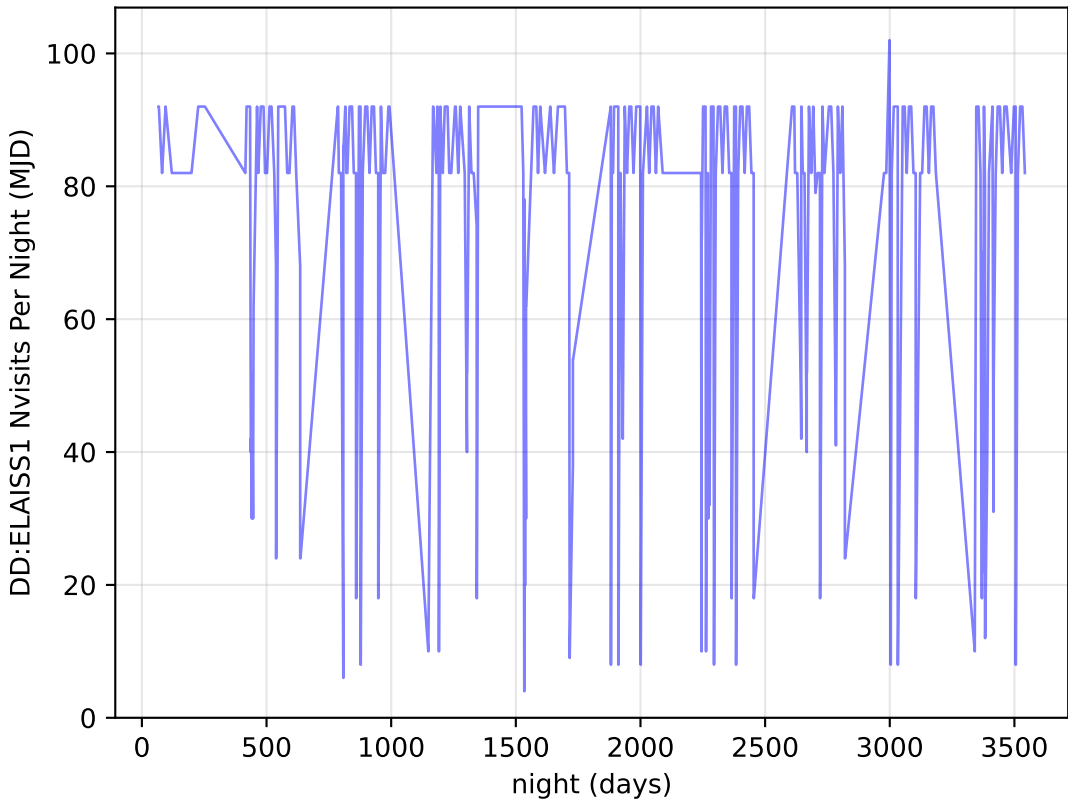
too_10_4v3.4_10yrs all bands: DD:ELAISS1 Nvisits Per Night
