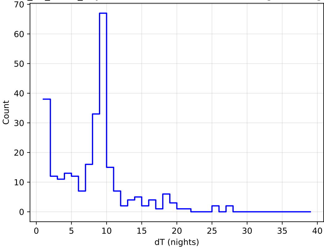
too_10_4v3.4_10yrs all bands: DD:ELAISS1 Delta Nights Histogram
